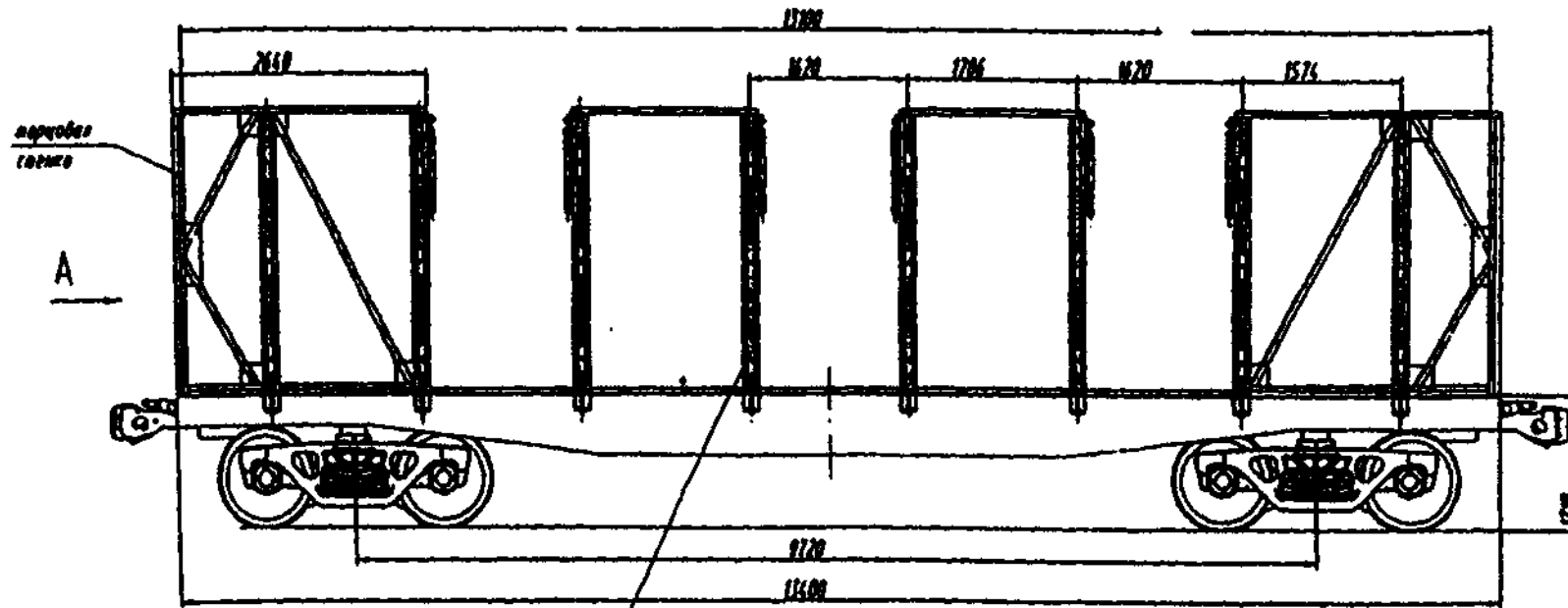
Промежуточная секция
